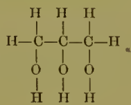
C_3H_8O_3 Glycerin (p. 18).
